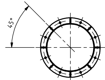
AF-AF ( 1 : 20 )
