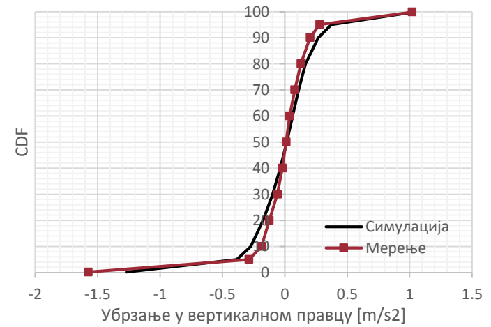
Слика 7-21. Убрзање сандука вагона у вертикалном правцу изнад водећег обртног постоља,
