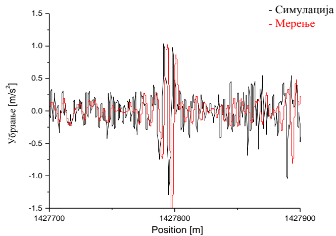
Слика 7-21. Убрзање сандука вагона у вертикалном правцу изнад водећег обртног постоља,
