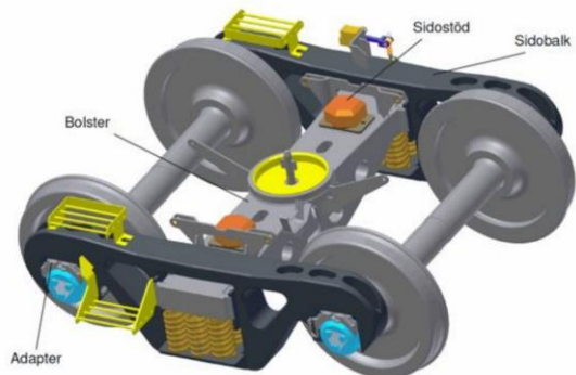
Слика 5-4 ASF Motion Control M976 тродено обртно постоље
