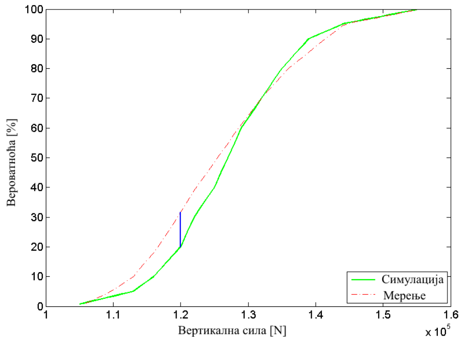
Слика 3-3. Колмоогов-Смирнова метрика
