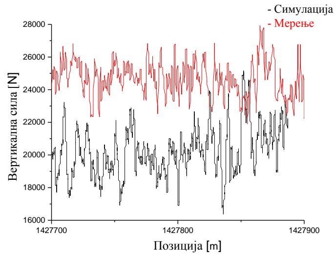
Слика 7-22. Вертикална сила у контакту точак-шина на спољашњем точку на водећој осовини на водећем обртном постољу, а) Сигнали добијени симулацијом и експерименталним испитивањем у просторном домену б) Кумулативне функције расподеле
