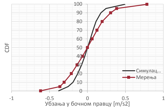
Слика 7-20. Убрзање сандука вагона у бочном правцу изнад водећег обртног постоља,
